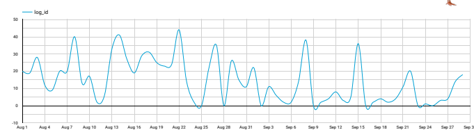
Aantal cases
